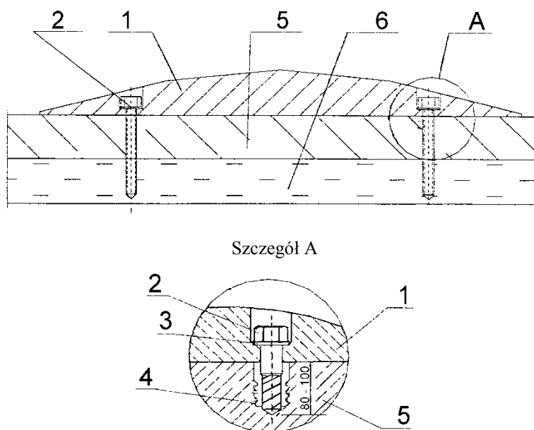
Rys. 4. Przykład umocnienia progu do nawierzchni jezdni
