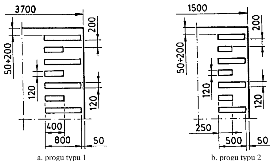
Rys. 2. Oznakowanie poziome
